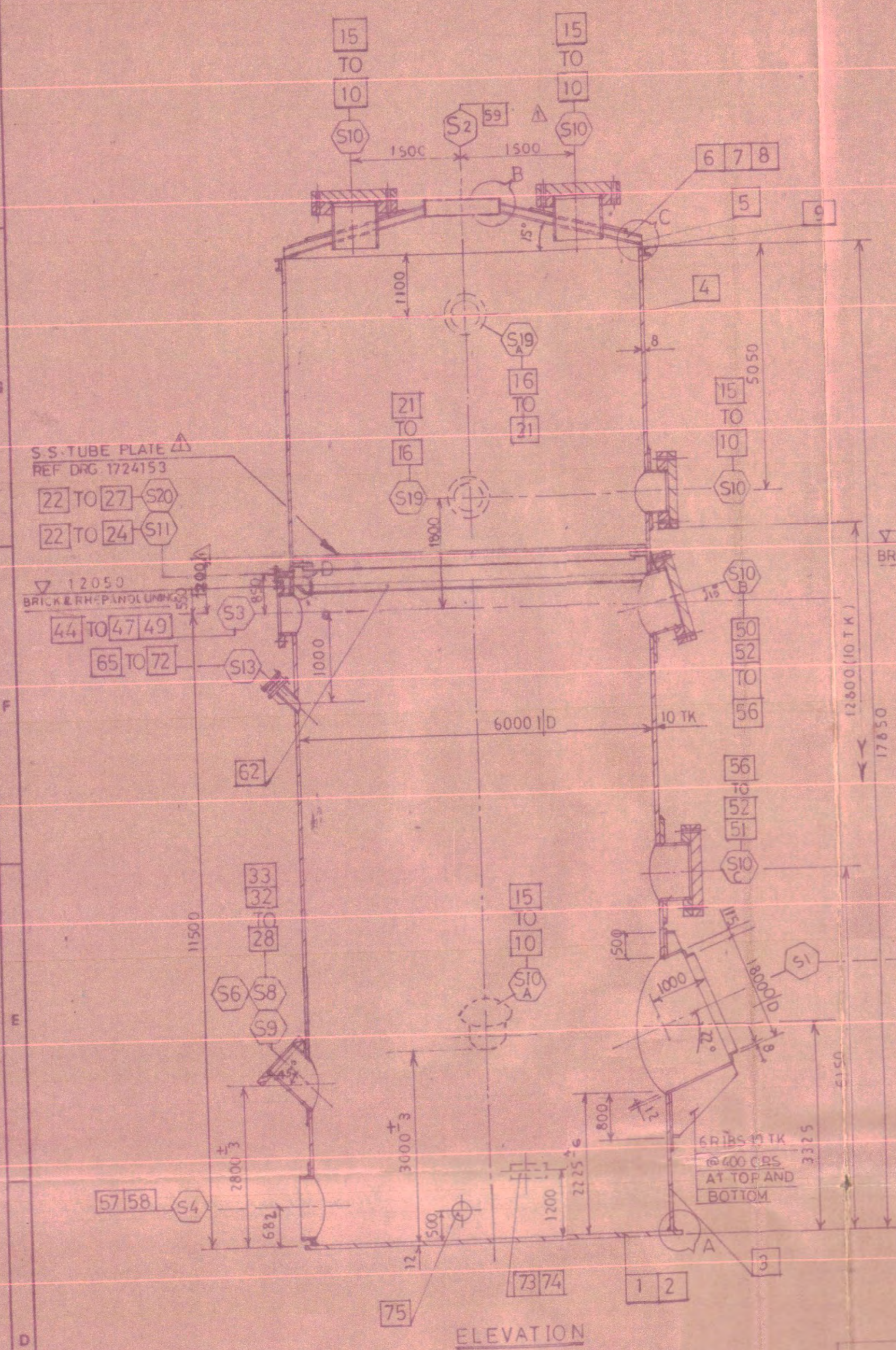
ELEVATION
